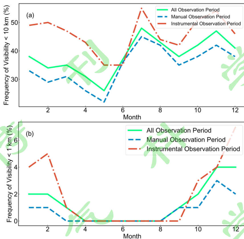
图 12 各时段北京站能见度<10km 频率(a) 月值, <1km 频率(b) 月值
