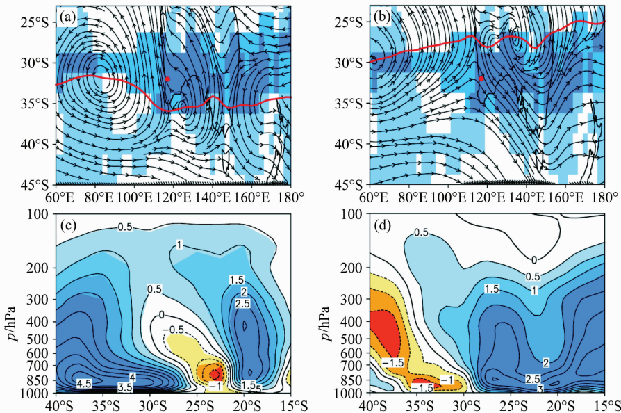
图 11 澳大利亚地区气候平均的 (a) 1 月和 (b) 7 月对流层中层 (925 hPa) 的水平环流 (红线: 副高脊线所在的位置; 红点: 西澳州首府 Perth 所在地; 阴影: 1 月和 7 月的风向变化至少超过 90° 的区域); 气候平均的 (c) 1 月和 (d) 7 月垂直速度的纬度—高度剖面 (纬向平均范围为 112.5°E~117.5°E) Fig. 11 The climatology stream lines at 925 hPa for (a) Jan and (b) Jul in Australia (red lines; the ridge lines of the subtropical high; red dot; the location of Perth; shadings; areas with the wind directions at least shifting 90° from Jan to Jul); latitude-pressure cross sections of the vertical velocity (averaged over 112.5°E~117.5°E) for (c) Jan and (d) Jul
