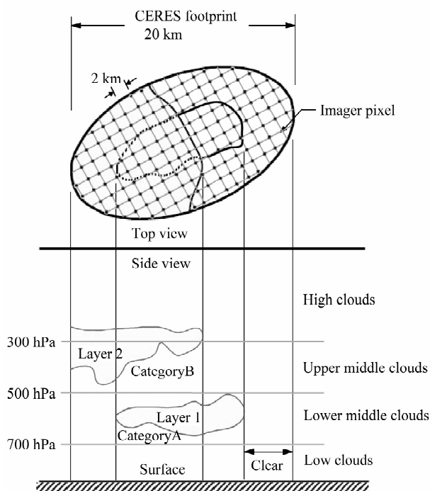
图 1 CERES 的空间分辨率和云的几何图形 (Geier et al., 2003)
