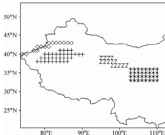
图 4 西北 4 个典型地域示意图
