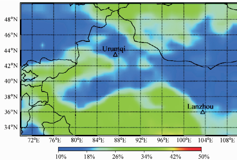
图 3 同图 2, 但为高层云量
