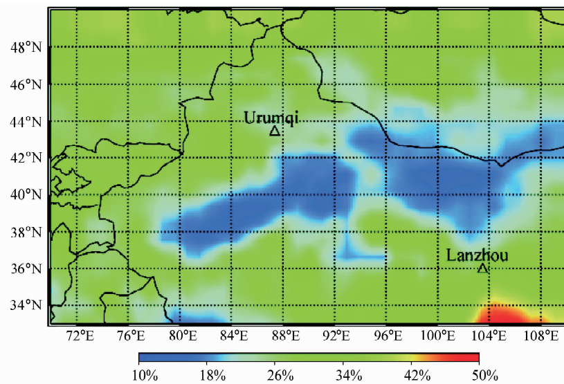
图 2 低层云量两年平均空间分布
