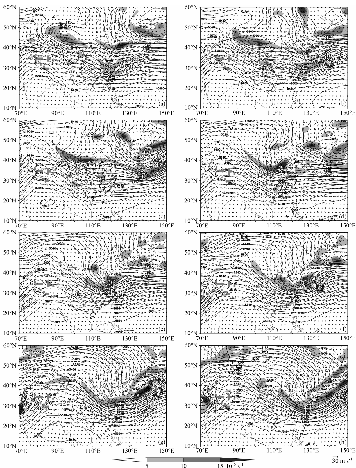
图 3 500 hPa 形势图，包括 500 hPa 涡度（阴影，单位： 10^{-5}\text{s}^{-1} ）、位势高度（实线，单位：gpm）、水平风场（箭头）和垂直速度（虚线，单位： 10^{-2}\text{m/s} ）：(a) 2004 年 12 月 28 日 12:00；(b) 29 日 00:00；(c) 29 日 12:00；(d) 30 日 00:00；(e) 30 日 12:00；(f) 31 日 00:00；(g) 31 日 12:00；(h) 2005 年 1 月 1 日 00:00。地形高度超过 5000 m 用小正方形填充，粗点线为槽线
