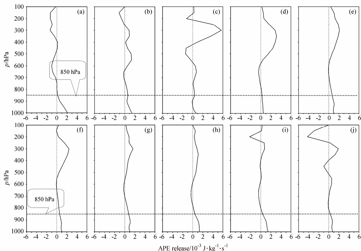
图7 大风区区域(图5中同时刻的虚线矩形框区域)平均的有效位能转化项垂直分布:(a) 2004年12月29日12:00;(b) 29日18:00;(c) 30日00:00;(d) 30日06:00;(e) 30日12:00;(f) 30日18:00;(g) 31日00:00;(h) 31日06:00;(i) 31日12:00;(j) 31日18:00
