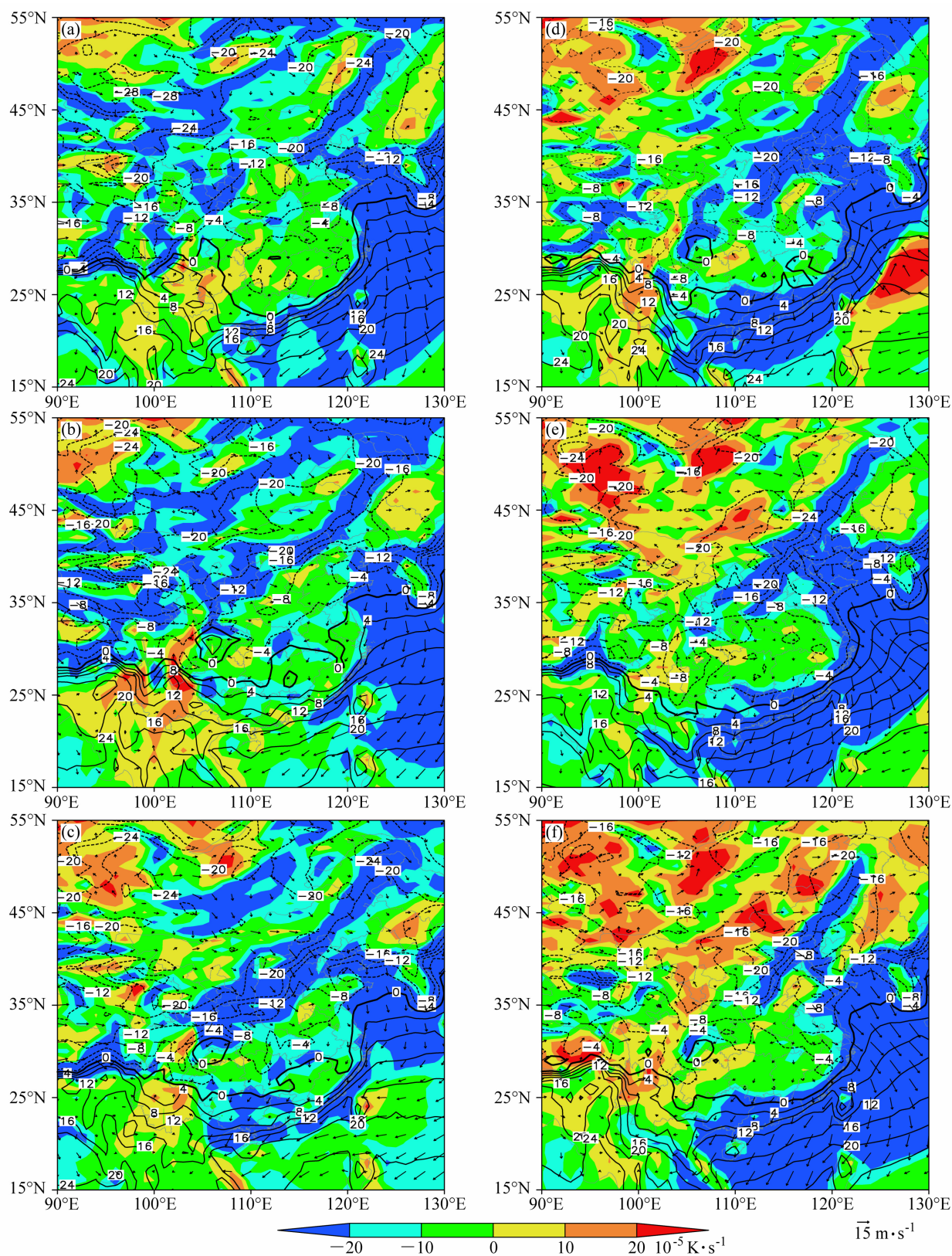
图2 地面温度场（等值线，单位：℃）、温度平流（阴影）和地面风场（矢量箭头）：（a）2004年12月29日00:00；（b）29日12:00；（c）30日00:00；（d）30日12:00；（e）31日00:00；（f）31日12:00
