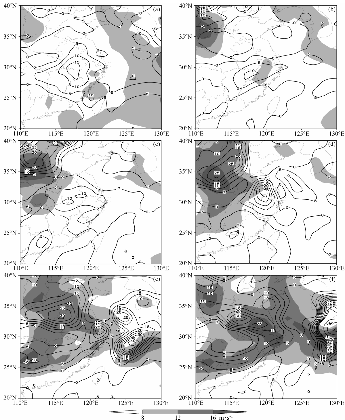
图6 有效位能转化图, 包括850 hPa风速大小 (阴影)、整层 (地面至100 hPa) 积分的有效位能向辐射散风的能量转化 (实线, 单位: \text{J m}^{-2} \text{s}^{-1} ): (a) 2004年12月29日12:00; (b) 29日18:00; (c) 30日00:00; (d) 30日06:00; (e) 30日12:00; (f) 30日18:00; (g) 31日00:00; (h) 31日06:00; (i) 31日12:00; (j) 31日18:00
