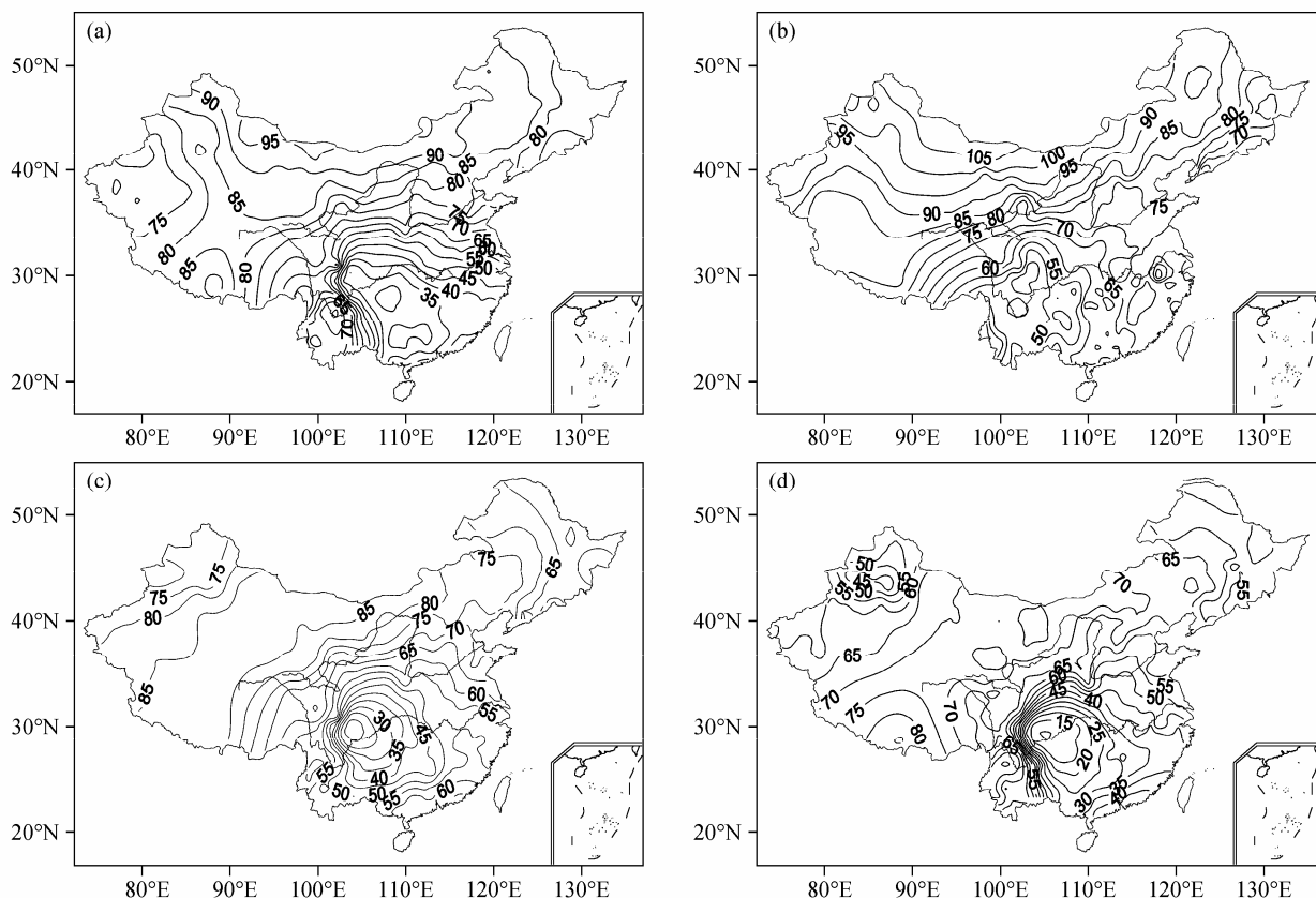
图3 春夏秋冬各季节平均日照时数(单位: 10 h)分布: (a) 春季; (b) 夏季; (c) 秋季; (d) 冬季
