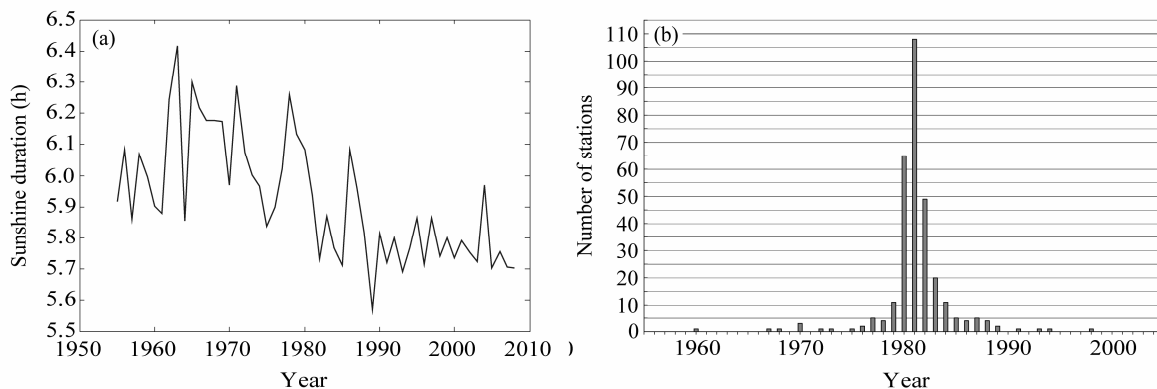
图4 中国地区区域平均后的(a)年日照时数时间序列与(b)各年份产生突变的观测站数
