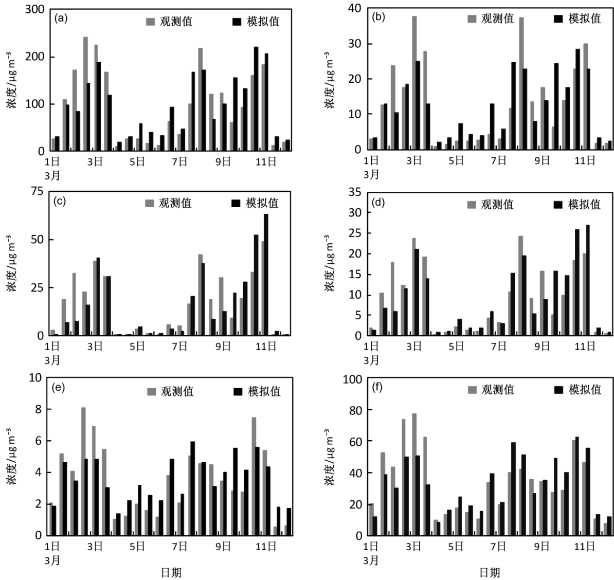
图4 2014年3月1~12日北京 (a) PM 2.5 、(b) SO 4 2- 、(c) NO 3 - 、(d) NH 4 + 、(e) BC、(f) OM 12 h 平均浓度模拟值 (Exp) 与观测值对比
