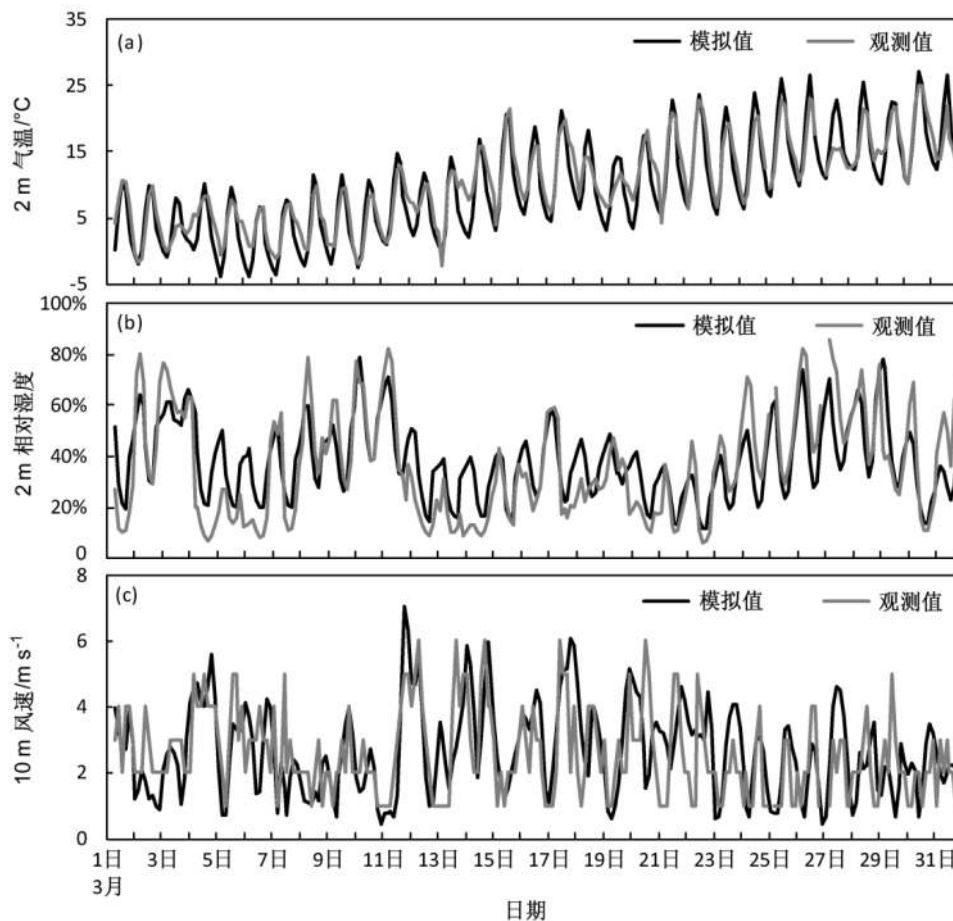
图 2 2014 年 3 月北京 (a) 2 m 气温、(b) 2 m 相对湿度和 (c) 10 m 风速观测和模拟值
