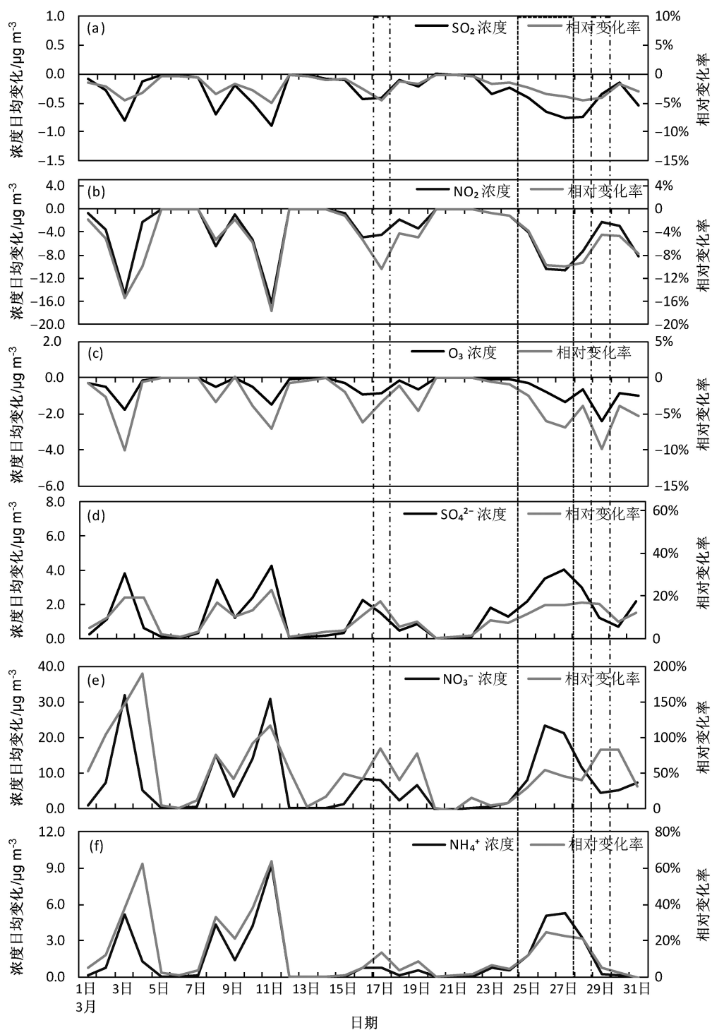
图7 模式模拟2014年3月北京非均相反应导致各物质浓度日均变化量 (Exp-Exp1) 和相对变化率 [(\text{Exp}-\text{Exp1})/\text{Exp1}]
