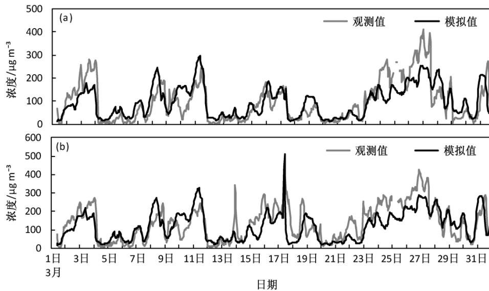
图3 2014年3月北京逐时(a) PM2.5、(b) PM10 质量浓度观测和模拟值(Exp)
