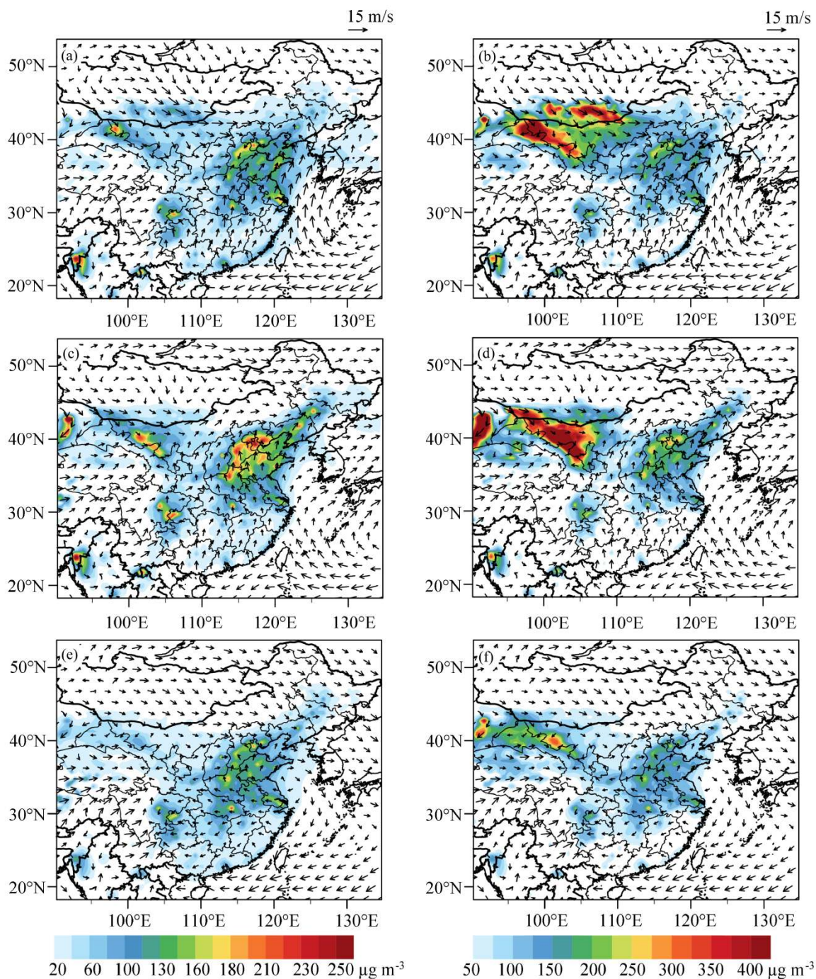
图 6 模式模拟的 (a、b) 沙尘期 (2014 年 3 月 16~17 日), (c、d) 霾期 (25~27 日) 和 (e、f) 月平均 PM 2.5 、PM 10 质量浓度和地面风场 (单位: \text{m s}^{-1} ) 空间分布
