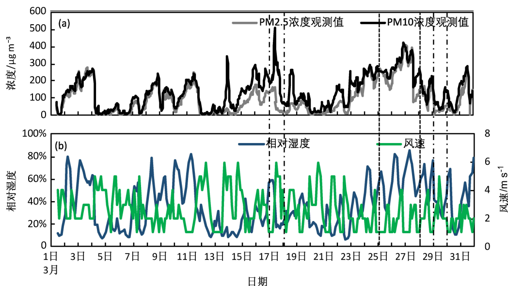
图 5 2014 年 3 月北京 (a) PM2.5、PM10 浓度观测值和 (b) 2 m 相对湿度、10 m 风速观测值
