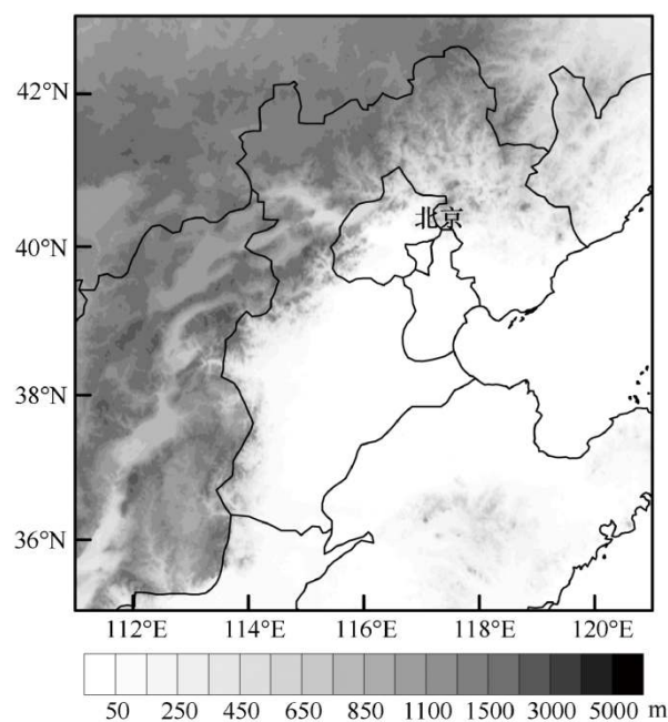
图 1 研究区域 (华北地区) 和地形
