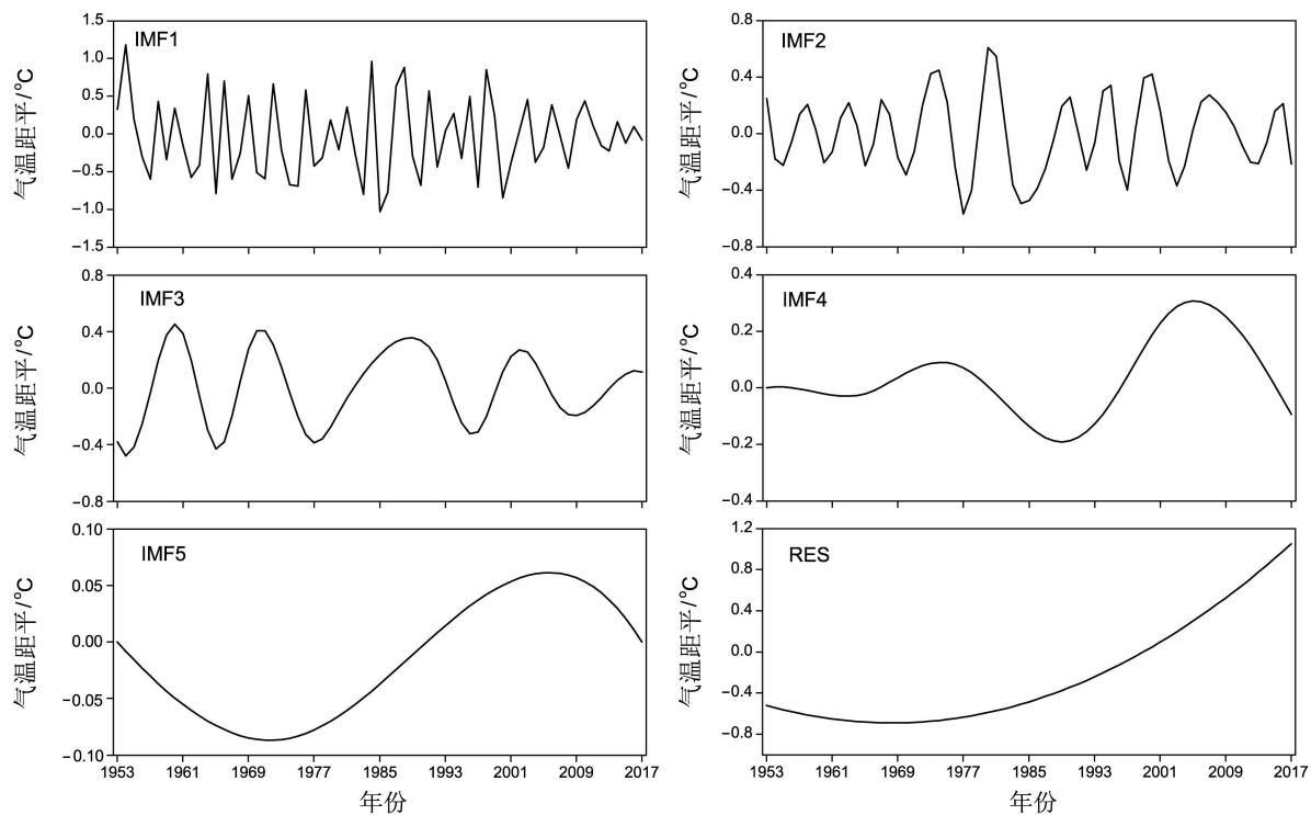
图4 1953~2017年黄河源区玛多站年平均气温距平序列经EEMD分解得到的5个IMF分量及趋势项(RES)
