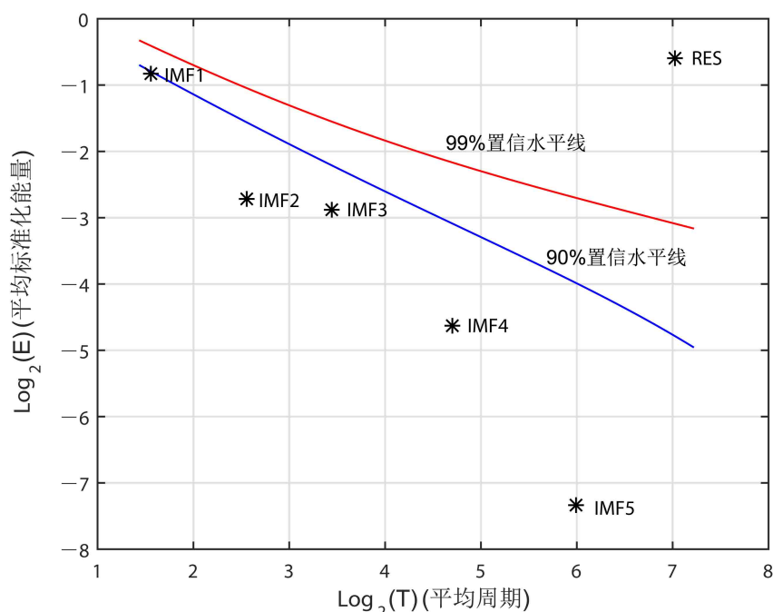
图5 1953~2017 年黄河源区玛多站年平均气温距平序列经 EEMD 分解的各分量信号的显著性检验
