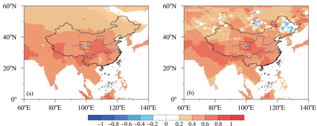
图 7 1953~2017 年 AMO 指数与 ( 0^{\circ}\sim 60^{\circ}\text{N} , 60^{\circ}\text{E}\sim 140^{\circ}\text{E} ) 范围内气温 (a) 原始序列和 (b) 65 a 以上时间尺度分量的相关系数空间分布 (点状阴影区表示相关系数通过 0.05 显著性水平)
