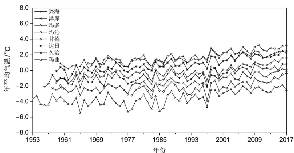
图2 黄河源区 8 个站点自建站以来年平均气温变化
