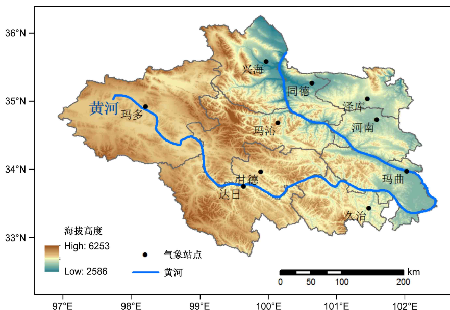
图 1 黄河源区气象站点的空间分布
