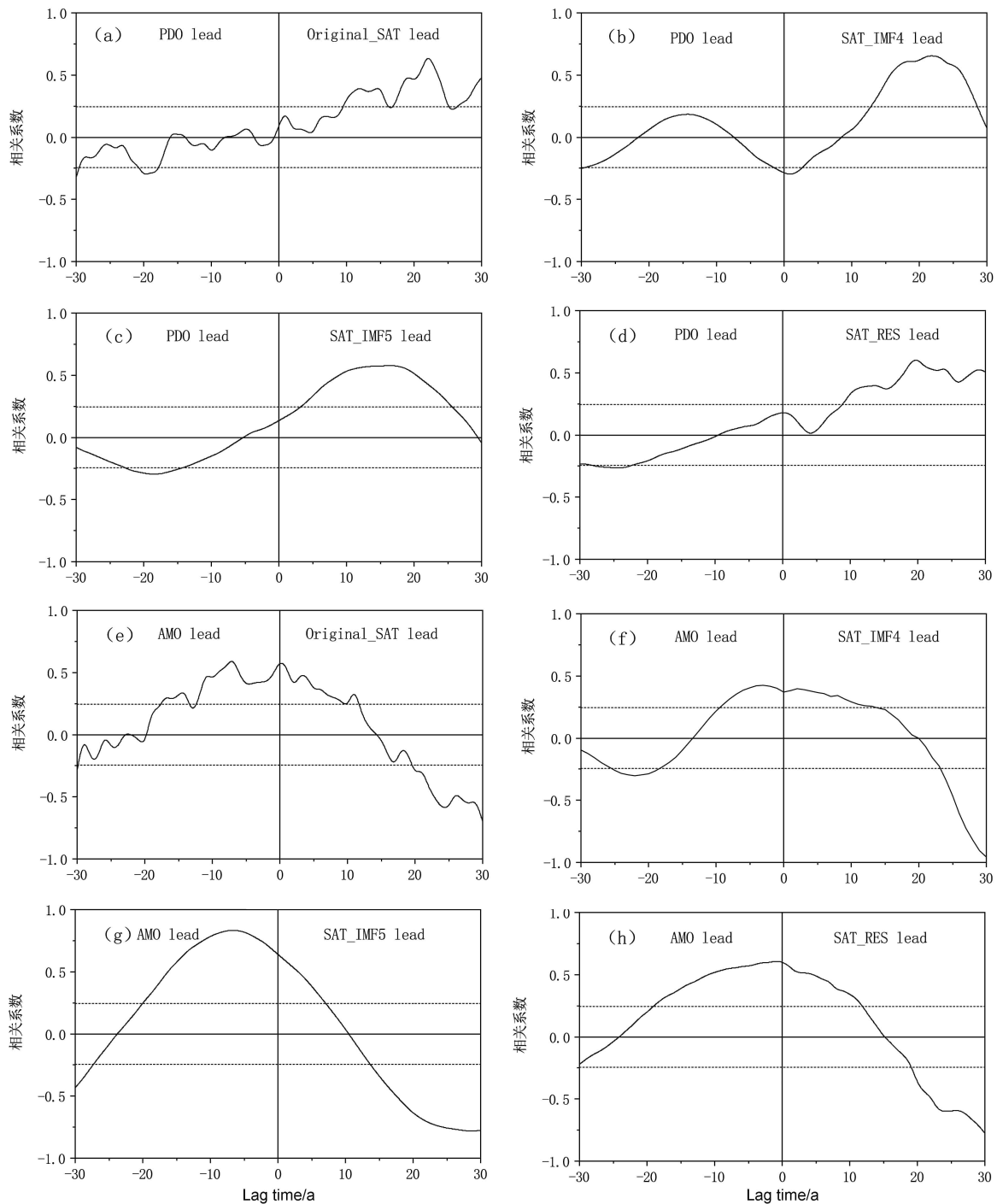
图6 1953–2017年黄河源区玛多站年平均气温距平序列及其3个年代际尺度以上分量与(a–d)PDO指数、(e–h)AMO指数的超前—滞后相关(横坐标为正值时表示气温超前,虚线表示相关系数通过0.05置信度水平):(a、e)年平均气温距平;(b、f)IMF4;(c、g)IMF5;(d、h)RES
