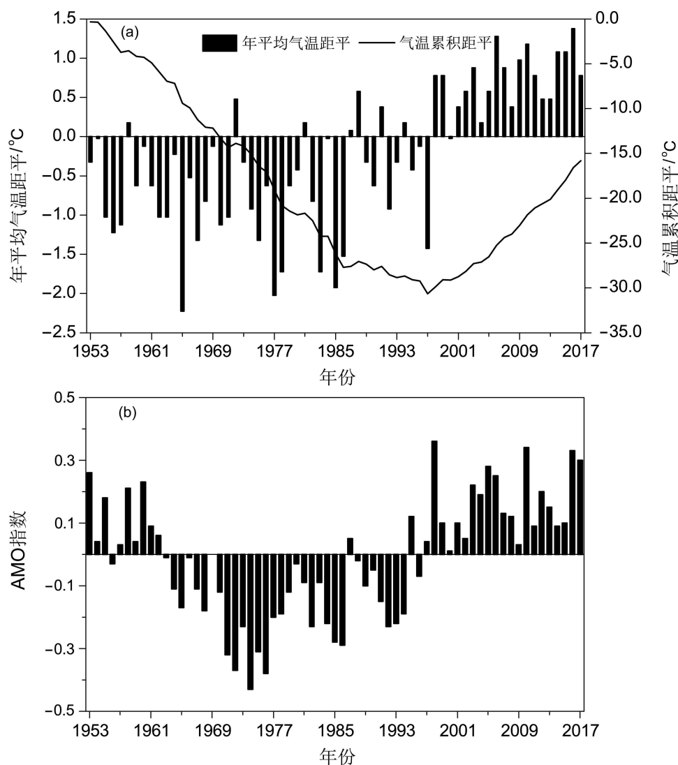
图3 1953~2017 年 (a) 黄河源区玛多站年平均气温距平历年变化及 (b) AMO 指数的时间序列
